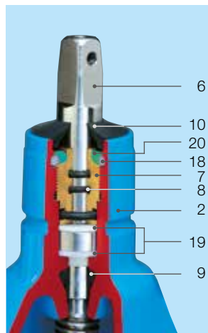
DN 50-200 Uloženie vretena na klzných podložkách
