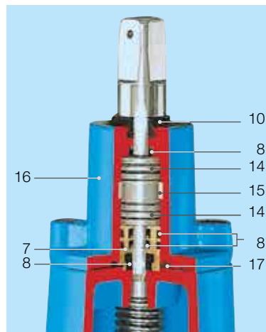
DN 250-600 Uloženie vretena na valivom ložisku
